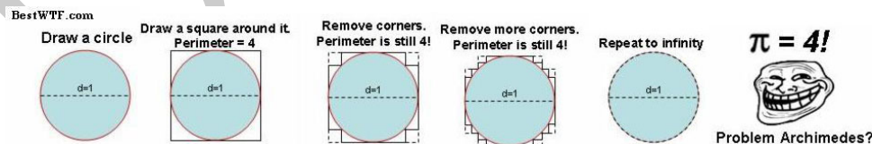
图 4.3.1: \pi = 4 的错误证明
