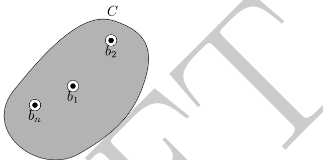
图 2.15.5: 留数定理
