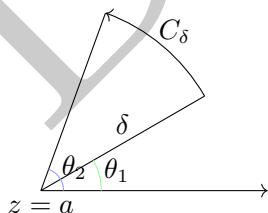
图 2.15.1: 小圆弧引理示意图
