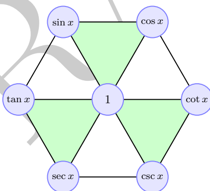
图 1.2.1: 同角三角函数助记图
